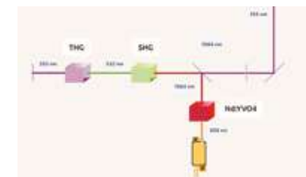
Схема генерации третьей гармоники
